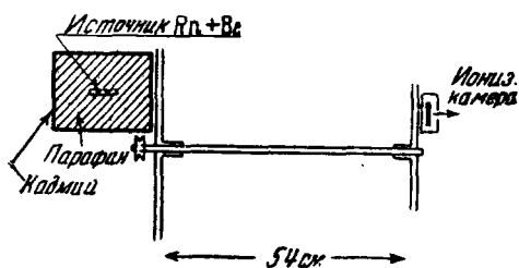
Рис. 1. Схема механического селектора Даннинга и др.
