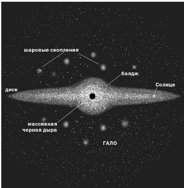
Рис. 3.19. Схематичное изображение Галактики.
