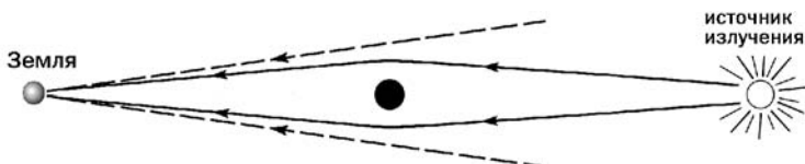
Рис. 1.15. Эффект линзирования.
