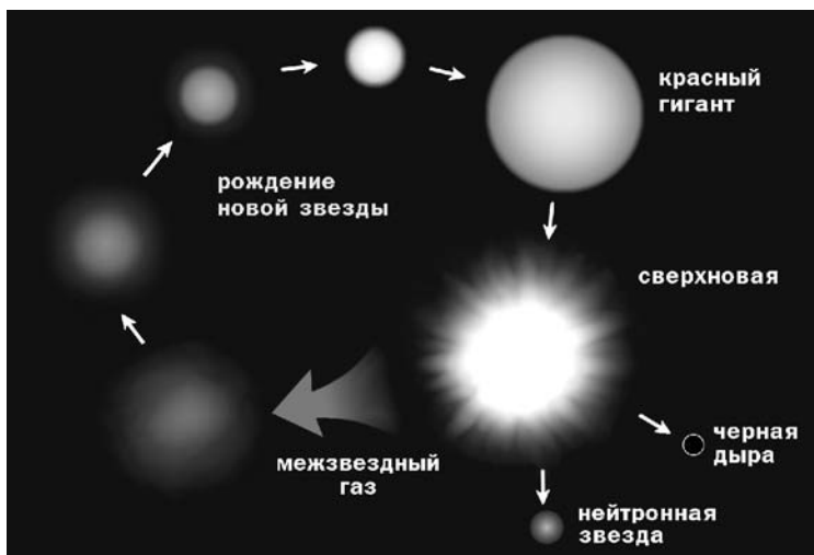
Рис. 3.4. Круговорот вещества в галактиках. Типичная молодая звезда рождается в газовом облаке, долго находится в квазистационарном состоянии, как наше Солнце сейчас, после исчерпания водорода переходит в стадию красного гиганта. Последний в конце концов взрывается, поставляя тяжелые элементы в окружающее пространство и пополняя газовые облака ядрами тяжелых химических элементов.
