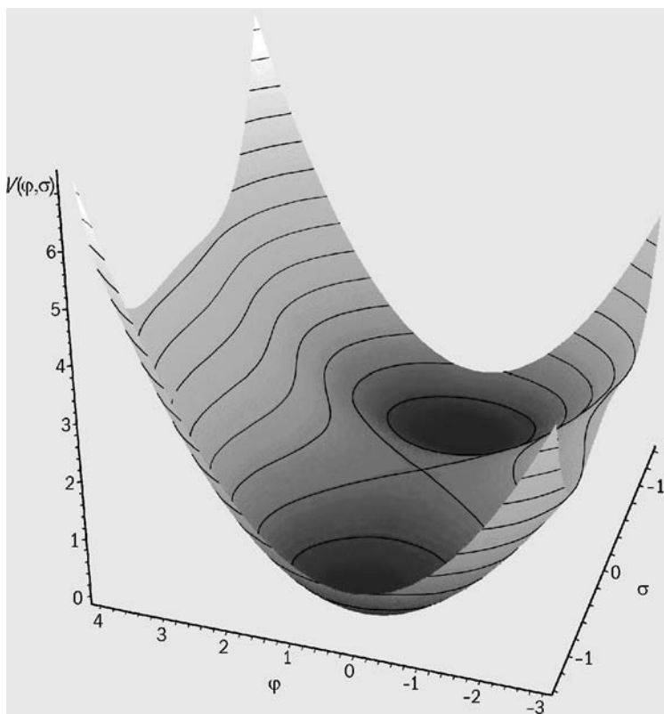
Рис. 1.7. Один из возможных потенциалов, используемых в космологии. Плотность энергии в определенной точке пространства (потенциал) зависит в данном случае от полей \phi и \sigma . Зависимость от нескольких гипотетических полей предоставляет дополнительные возможности для объяснения происхождения такой вселенной, как наша.
