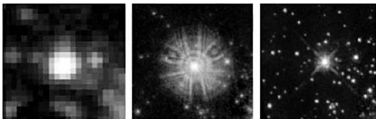
Рис. 4.5. Так видели астрономы звезду Мельник-34. Слева — наилучшее изображение звезды с наземной обсерватории, в середине — та же звезда, сфотографированная телескопом «Хаббл» до юстировки оптики, справа — после.
