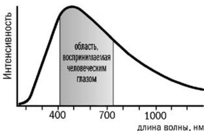
Рис. 1.9. Зависимость интенсивности излучения с поверхности Солнца (ее температура составляет приблизительно 5 700 К) от длины волны. Интенсивность — число фотонов, излученных в секунду.
