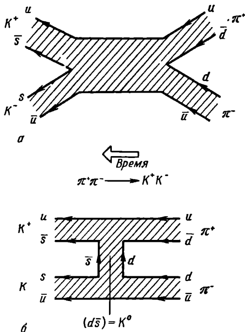
Рис. 13.6. Процесс обмена одним каоном между двумя мезонами.
