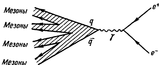
Рис. 13.8. Диаграмма для процесса столкновения электрона с позитроном.
