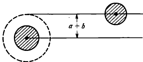
Рис. 13.1. Столкновение шаров с радиусами a и b .
