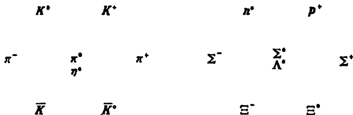
Рис. 7.1. Семейство мезонов.
