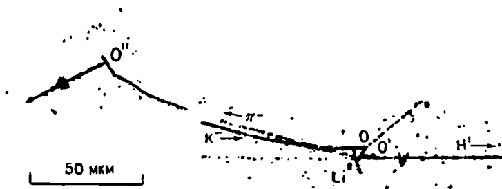
Рис. 6.1. Треки частиц в фотоэмульсии. (Фото проф. Леви-Сетти из журнала «Нуово чименто».)
