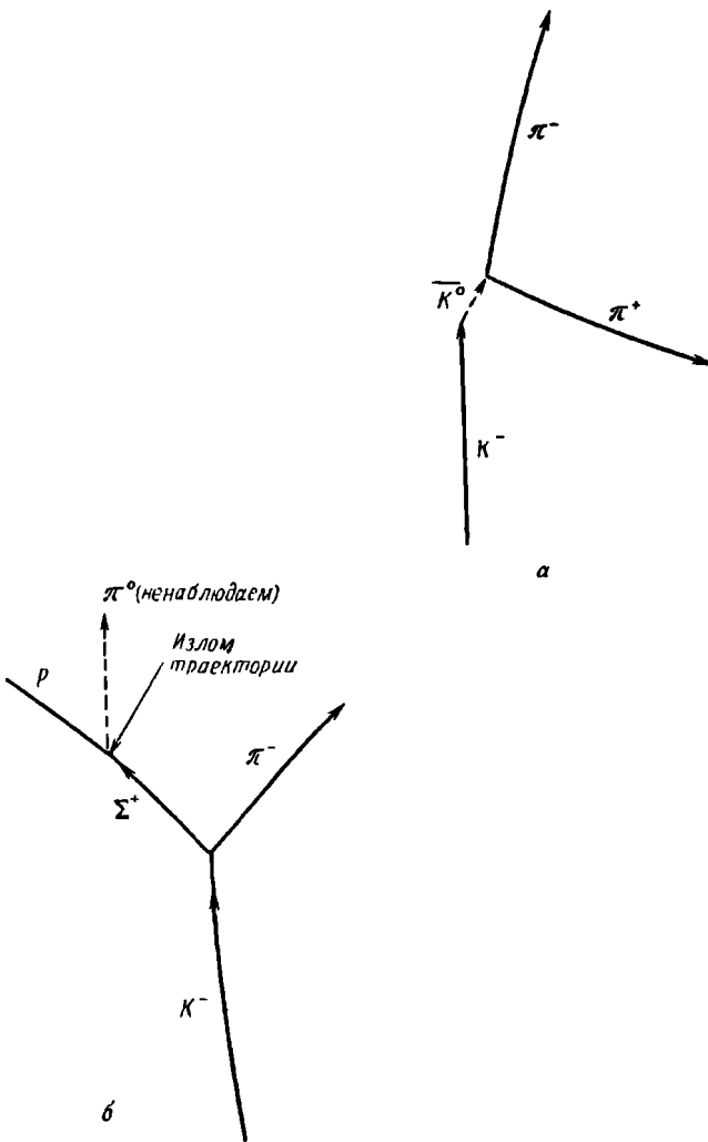
Рис. 3.2. Фотография следов заряженных частиц в пузырьковой камере, облучаемой пучком K^- -мезонов. На чертеже нарисованы присутствующие на фотографии треки, соответствующие двум конкретным процессам столкновения K^- -мезонов с наполняющими камеру протонами. (Снимок любезно предоставлен проф. Леви-Сетти.) a —рождение и распад K^0 : K^- + p \rightarrow n + \bar{K}^0 ; \bar{K}^0 \rightarrow \pi^+ + \pi^- ; b —рождение и распад \Sigma^+ : K^- + p \rightarrow \Sigma^+ + \pi^- ; \Sigma^+ \rightarrow p + \pi^0 .
