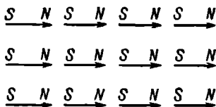
Рис. 17.1. Ферромагнетизм. Направления всех атомных магнитов одинаковы.
