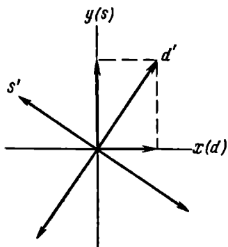
Рис. 18.1. Поляризация и кварки d , s , d' , s' .
