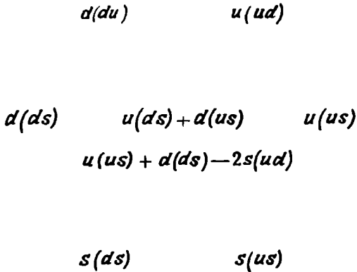
Рис. 10.2. Построение барионного октета:
