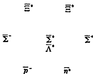
Рис. 7.3. Семейство антибарионов.
