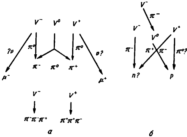
Рис. 7.5. а — V-частицы, интерпретируемые как мезоны; б — V-частицы, интерпретируемые как барионы.
