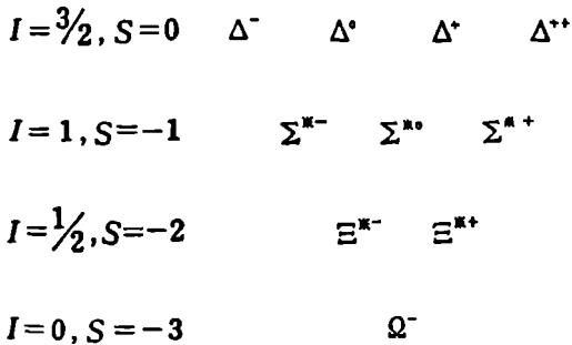
Рис. 10.3. Барионный декуплет.
