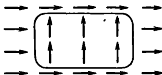
Рис. 17.2. Спонтанное нарушение симметрии: локальное разупорядочение.
