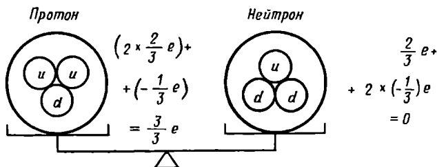
Рис. 3.1. Протон и нейтрон.
