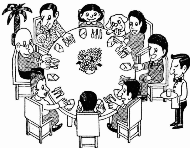
Спонтанное нарушение симметрии: пример Салама.
