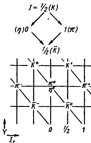
Рис. 7.4.
