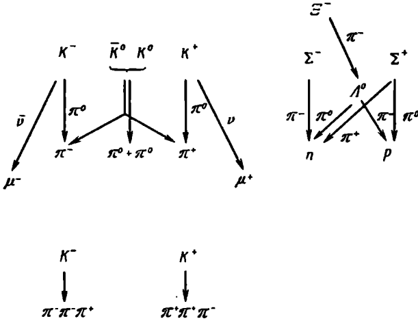
Рис. 7.6.
