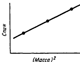
Рис. 13.2. Траектория Редже.
