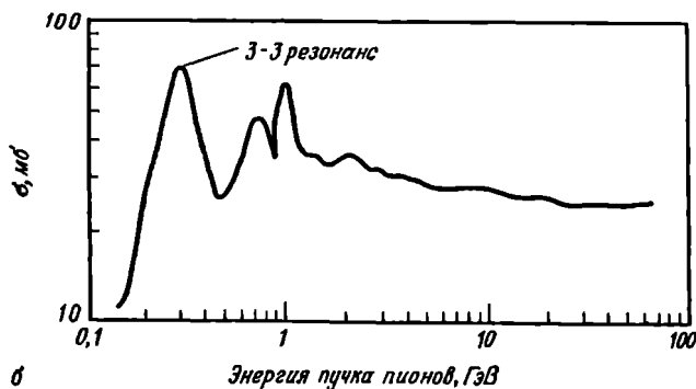
Рис. 7.7. Резонансное рассеяние пионов на нуклонах ( \pi N -рассеяние): а—полное сечение процесса \pi^+ p ; б—полное сечение процесса \pi^- p . 1 \text{ мб} = 10^{-27} \text{ см}^2 .
