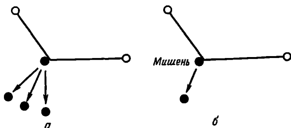
Рис. 14.1. Неупругое (а) и упругое (б) рассеяние.
