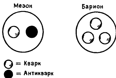
Рис. 2.1. Мезоны и барионы.
