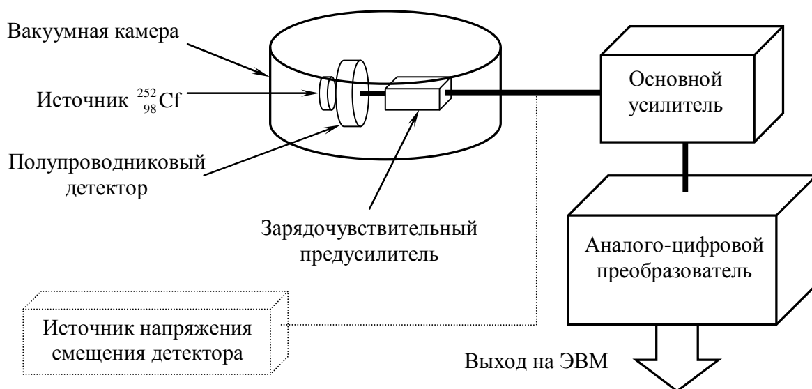
Рис. 1: Блок-схема установки для измерения спектра осколков деления.
