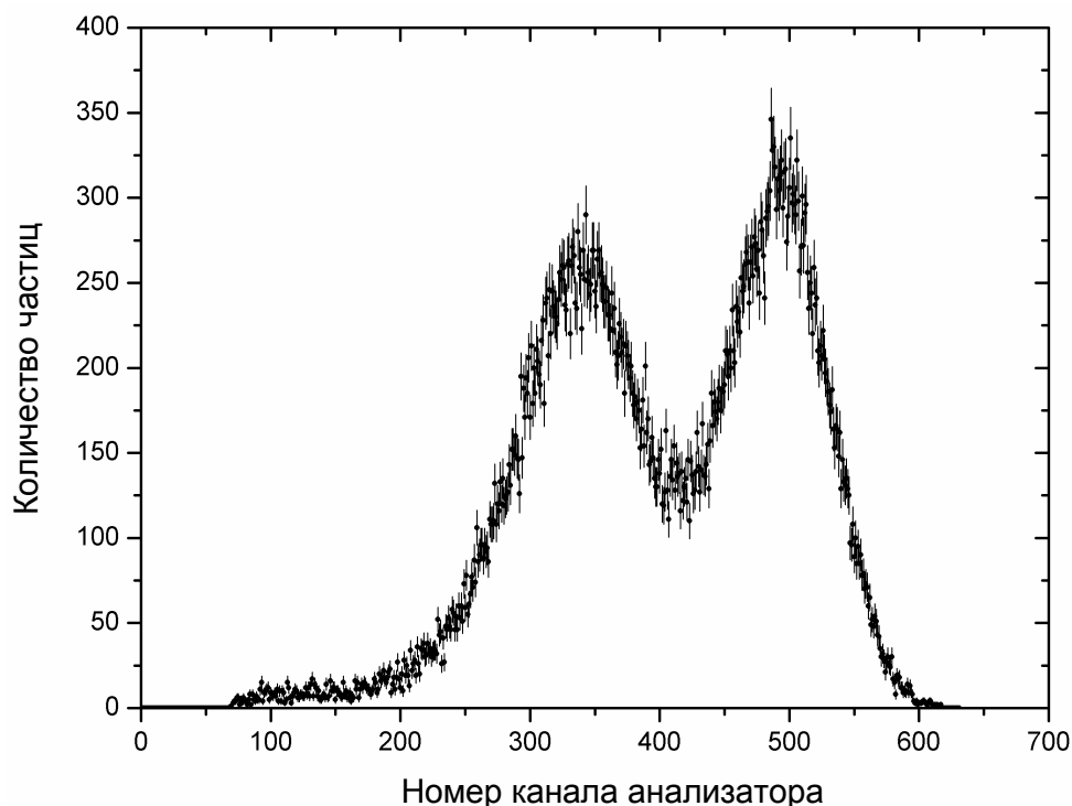
Рис. 3: Спектры осколков спонтанного деления ^{252}_{98}\text{Cf} . Время набора около 6 часов.
