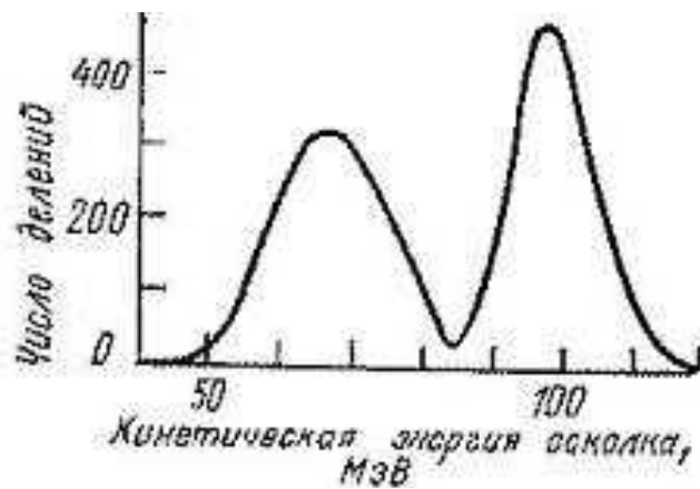
Рис. 10: Распределение по энергии осколков деления {}^{235}_{92}\text{U} тепловыми нейтронами
