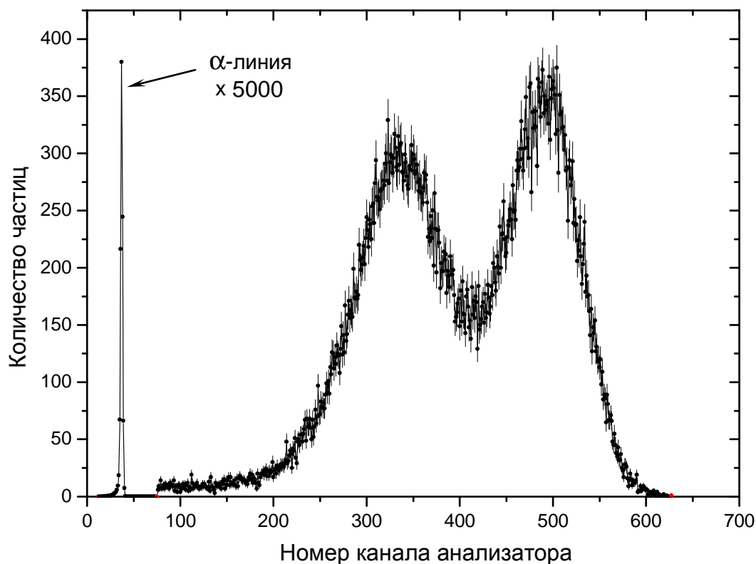
Рис. 2: Спектры осколков спонтанного деления и \alpha -частиц ^{252}_{98}\text{Cf} . Число отсчетов в спектре \alpha -частиц уменьшено в 5000 раз для возможности сравнения. Время набора около 6 часов.
