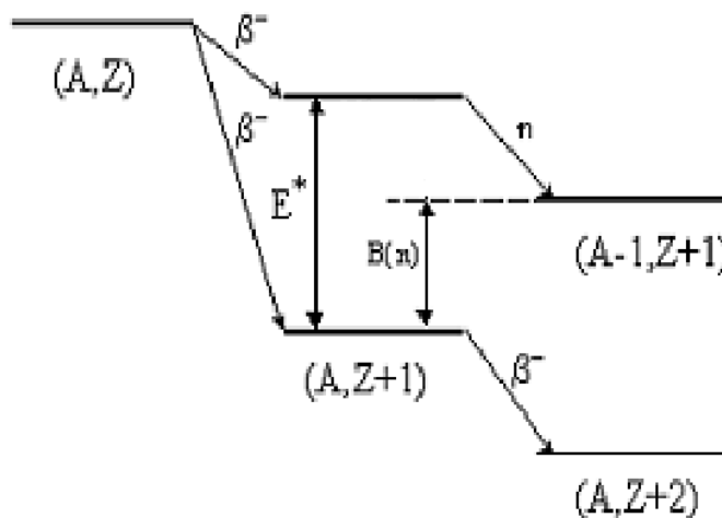
Рис. 11: Схема образования запаздывающих нейтронов: E^* – энергия возбуждения ядра (A, Z + 1) ; B(n) – энергия отделения нейтрона в ядре (A, Z + 1) ; E_n – кинетическая энергия запаздывающего нейтрона
