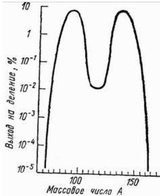
Рис. 9: Массовое распределение осколков деления {}^{235}_{92}\text{U} тепловыми нейтронами
